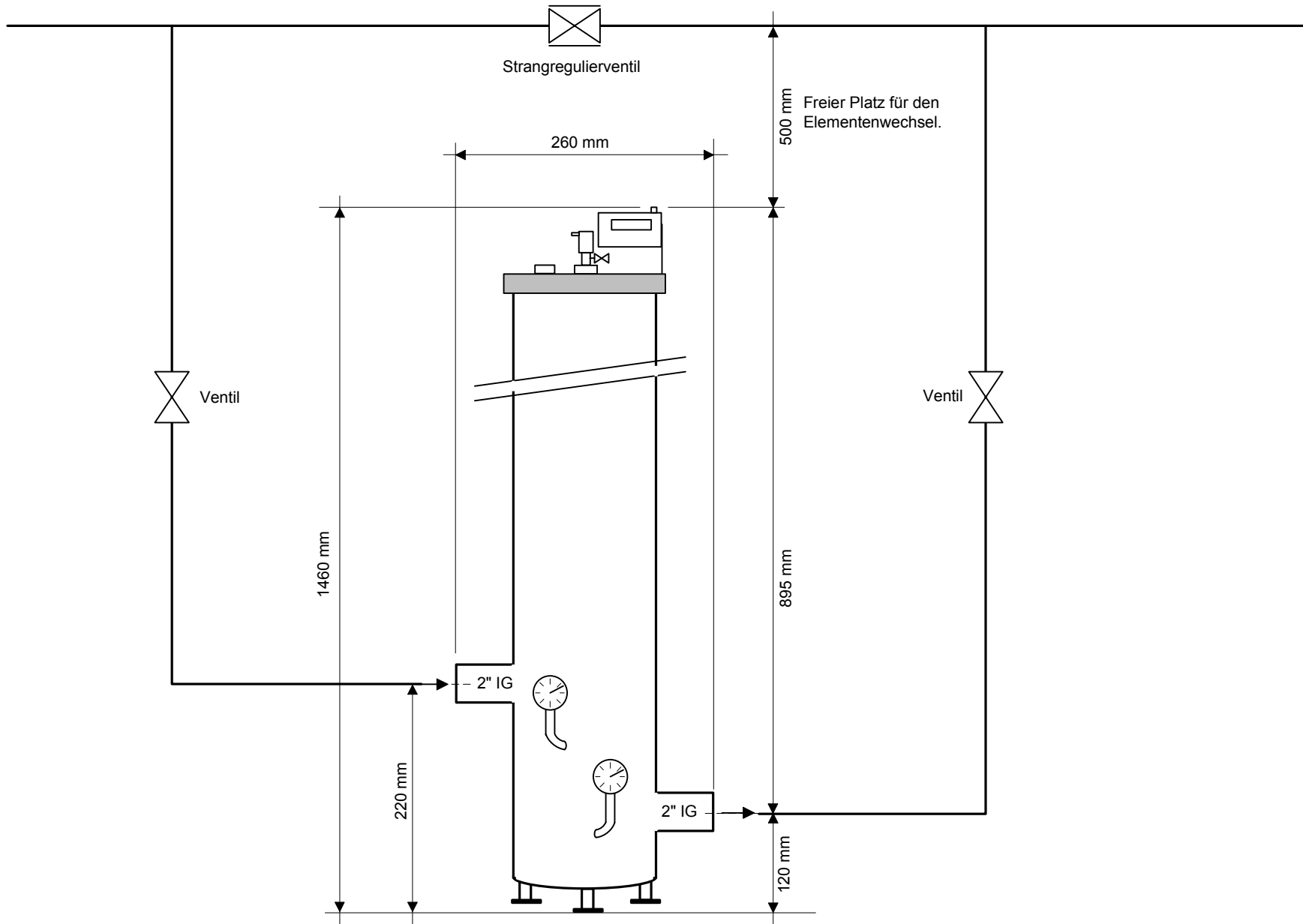
Teilstromfiltration
